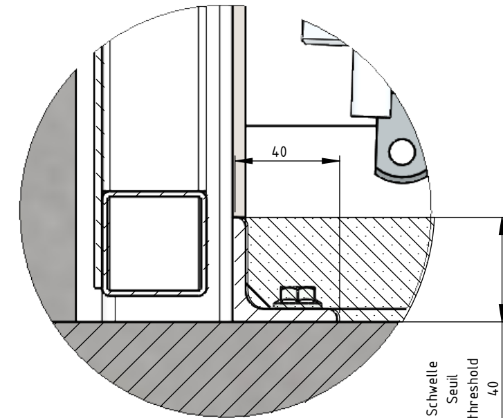
DETAIL D 1 : 2
