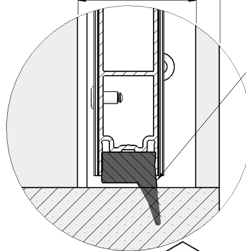
DETAIL B MAßSTAB 1 : 1
