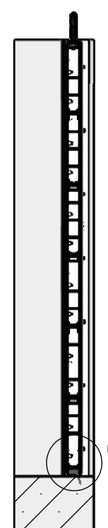
SCHNITT A-A
