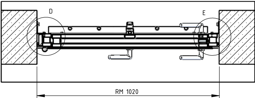
SCHNITT B-B
